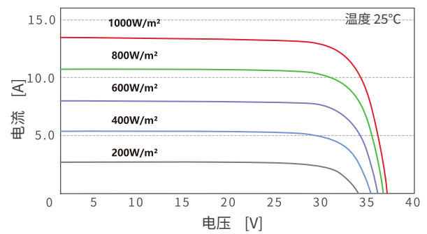
组件的I-V曲线
